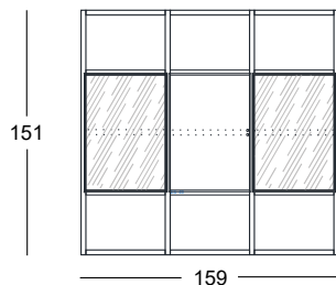
ESTANTERIA N°1 159X151X35 COMPOSICION N°32
