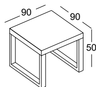
MESA CENTRO 90 X 90 X 50
