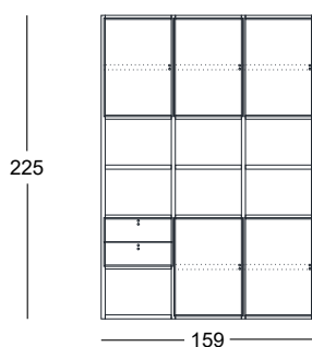
ESTANTERIA N°2 159X225X35 COMPOSICION N°30
