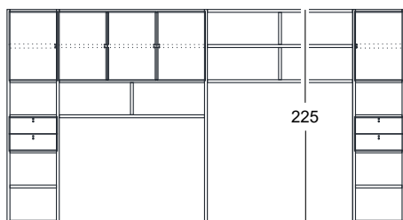
ESTANTERIA N°3 419X225X35 COMPOSICION N°31
