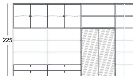
ESTANTERIA N°4 369X225X35 COMPOSICION N°33
